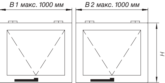
PRIMAT-A, тип: hm, 2 Створки рядом
