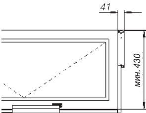
PRIMAT-A электропривод сбоку SM 100 или EM 100
