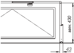
PRIMAT-FL 190 электропривод сбоку SM 100 или EM 100
