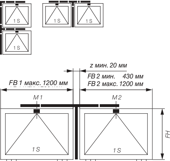
PRIMAT-FL 190, Тип: hm, 2 Створки рядом
