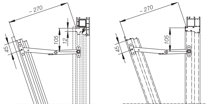
Фальцевые ножницы на окне из пластика и из лёгкого металла
