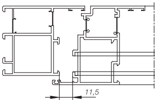
Прикручиваемая пластина для LM фурнитурного паза 16 мм
