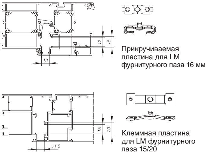
Фальцевые ножницы на окне из пластика и из лёгкого металла
