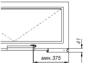
PRIMAT-A электропривод снизу SM 100 или EM 100
