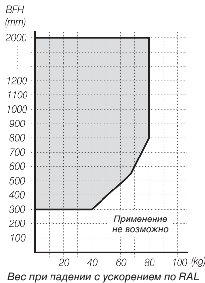
Диаграмма применения для фальцевых ножниц, применение парами.
