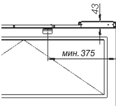
PRIMAT-FL 190 электропривод сверху SM 100 или EM 100
