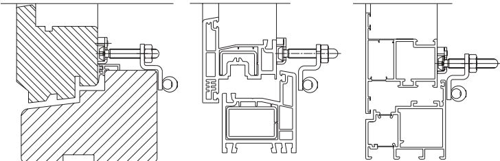
Вертикальные сечения на окнах из дерева, пластика и металла
