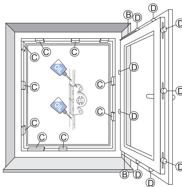
Наглядная схема мест смазки
