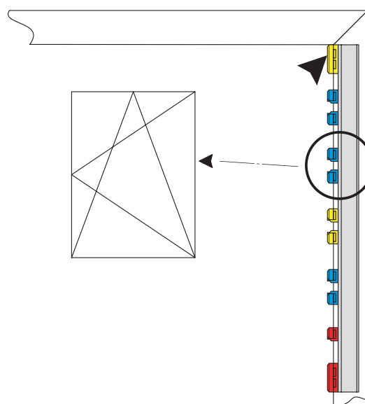
Ответные планки с петлевой стороны
