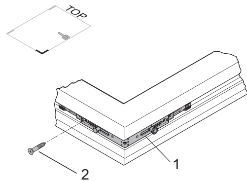
Угловая передача E1.PA
