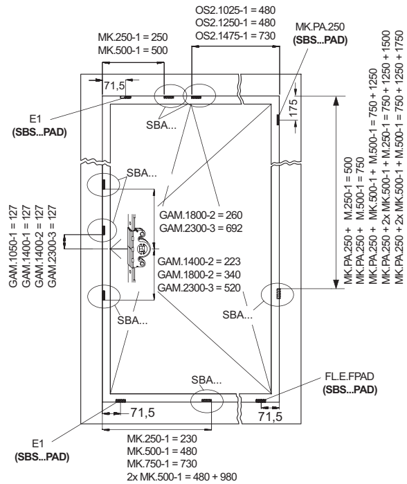
Места установки ответных планок DK "центральное положение ручки"
