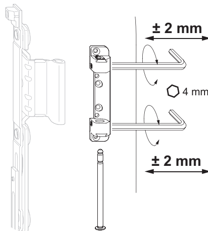
Регулировка на верхней петле
