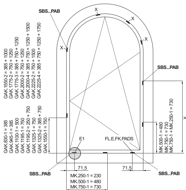
Места установки ответных планок "фиксированное положение ручки" X = размер согласно чертежу
