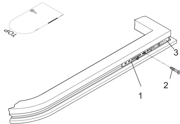
Блокада МК
