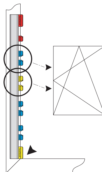
Ответная планка SBA... для ГАК, устанавливается вертикально
