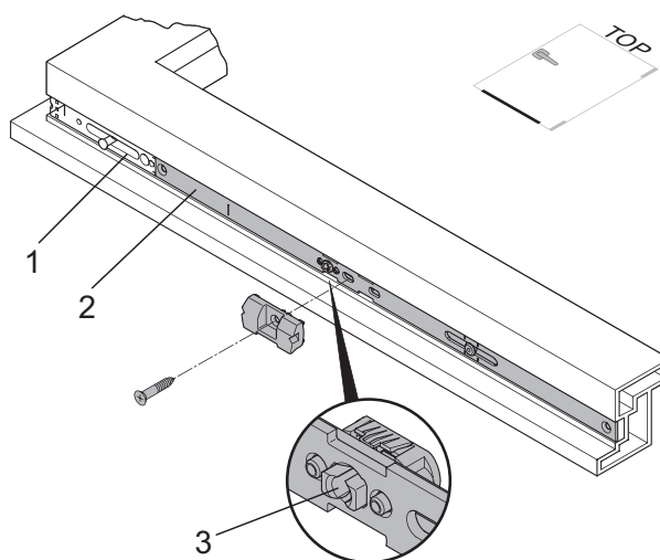
Трамплин AL.M.F12
