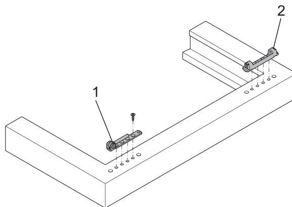
Верхняя петля и нижняя петля
