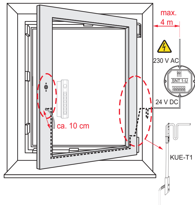
Каблирование створки
