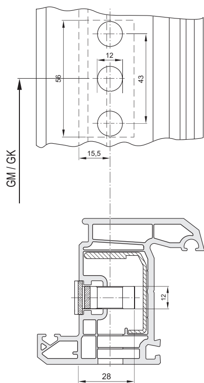
В-3-1: Сверление и фрезеровка GAK/GAM ...D = 15,5 мм
