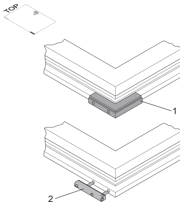
Петля на створку FK
