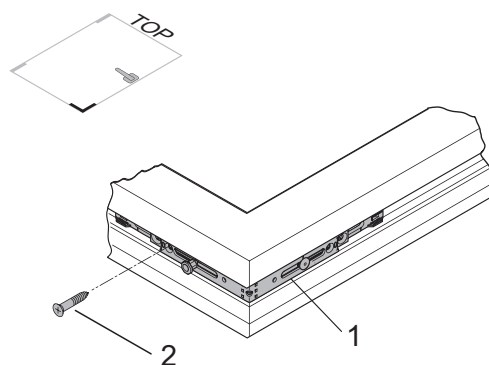
Угловая передача E1
