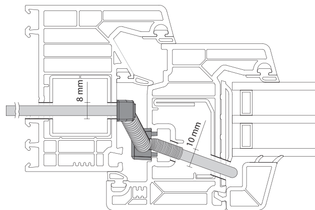
Чертеж по монтажу: соединитель кабеля FFK = край фальца створки RFK = край фальца рамы
