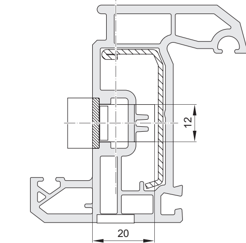
V-3-2: Сверление и фрезеровка GAK/GAM ..D = 7,5 мм
