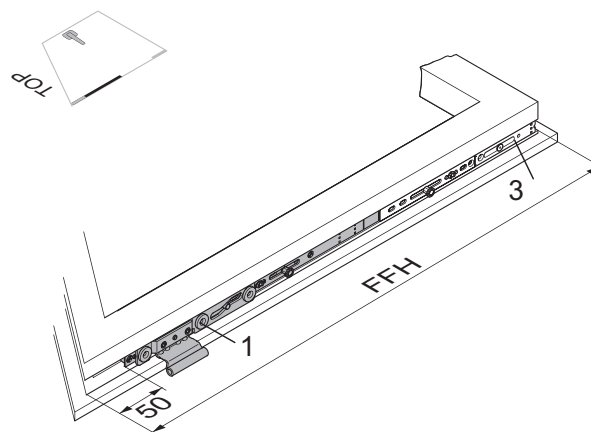
Петля DL.PADS
