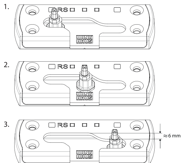
Функция SBS.K.PAB...PAS
