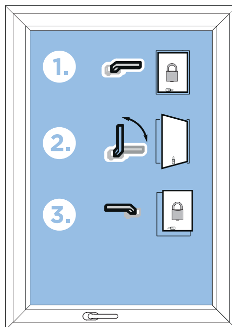
activPilot Comfort PAD (ручка на нижней части створки)
