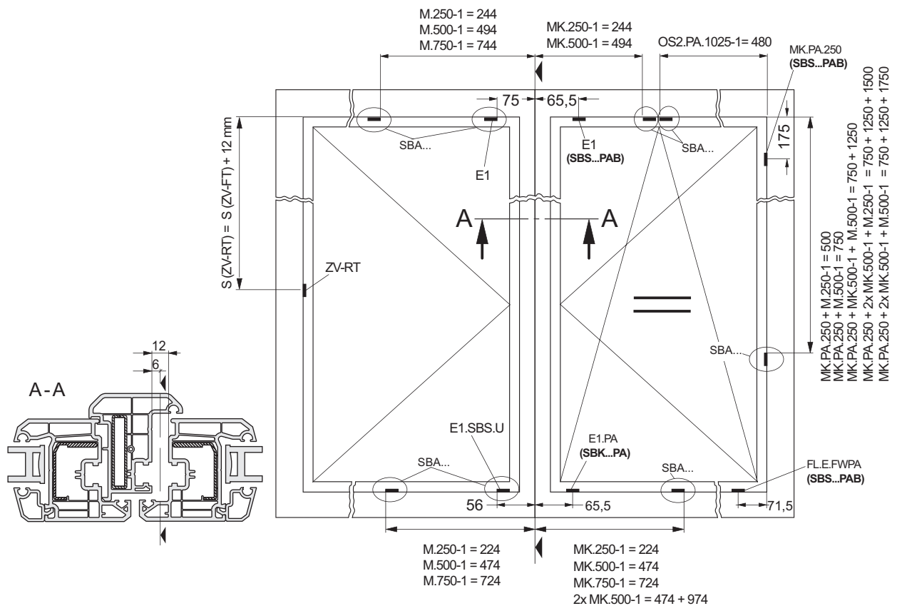
Места установки ответных планок для поворотного и поворотно-откидного штапелевого окна
