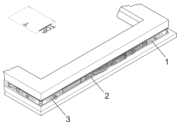
Верхняя шина OS2.PA...
