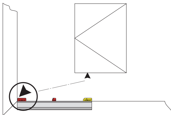
SBS...PAD (устанавливается внизу)
