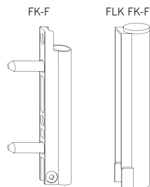
Юстировочный винт для регулировки композитной втулки
