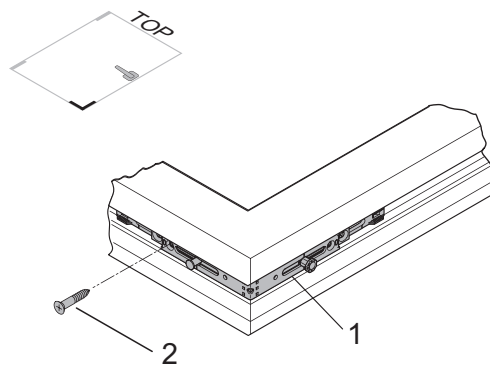
Угловая передача E1.PA
