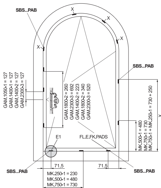
Места установки ответных планок "центральное положение ручки" X = размер согласно чертежу
