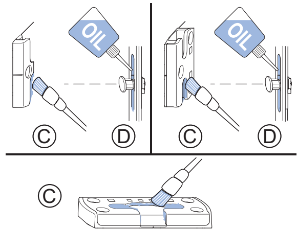
Места смазки
