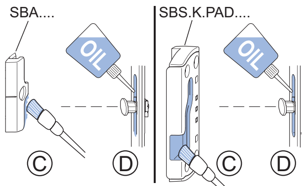
Ответные планки
