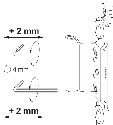
Регулировка на петле
