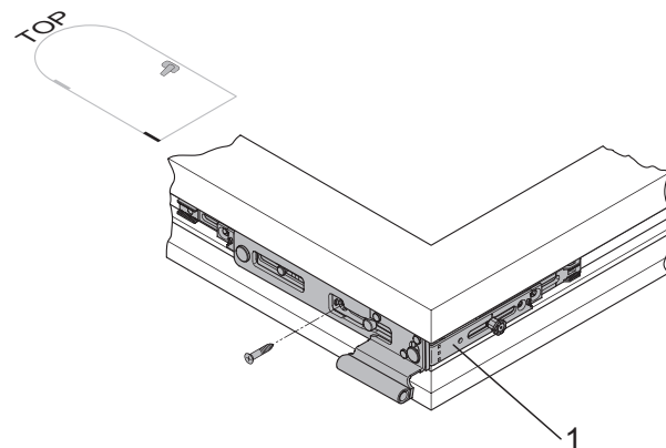
Петля на створку FL.E...PA..
