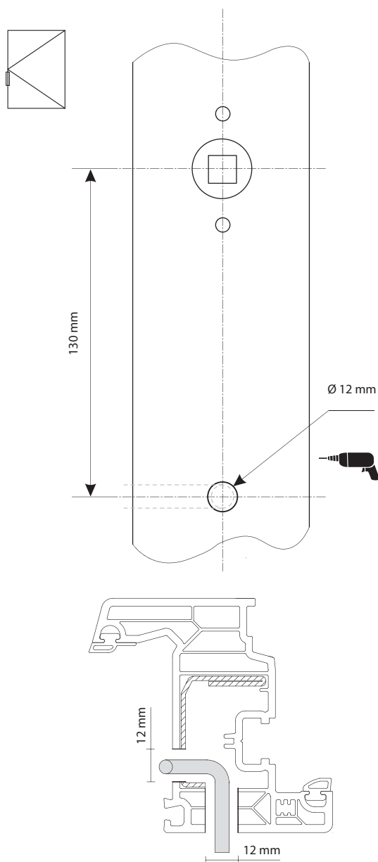
Прокладка кабеля от мотора
