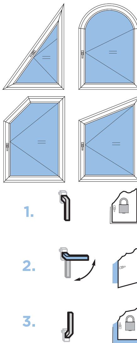
activPilot Comfort PADS - открывание и параллельное смещение оконных створок нестандартных форм
