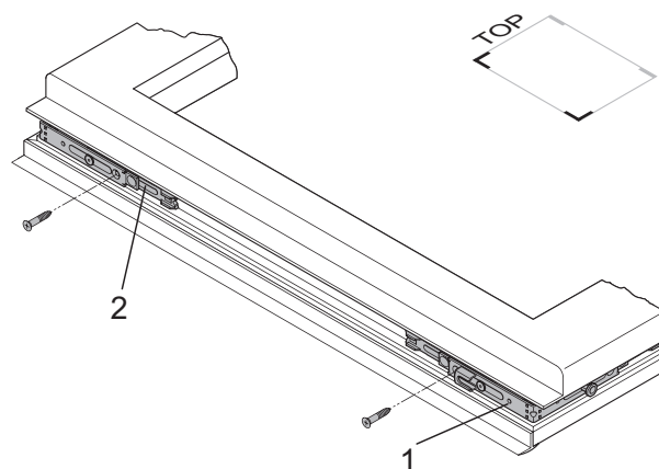
Угловая передача E1 (1) / E1.SBS.U (2)
