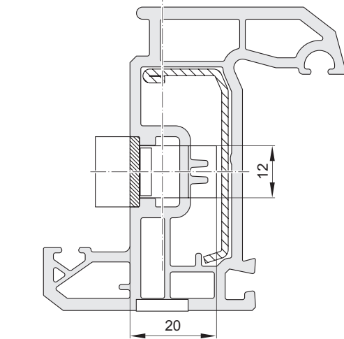
B-3-2: Сверление и фрезеровка GAK/GAM ..D = 7,5 мм
