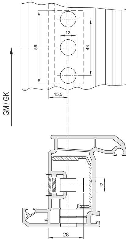
B-3-1: Сверление и фрезеровка GAK/GAM ...D = 15,5 мм
