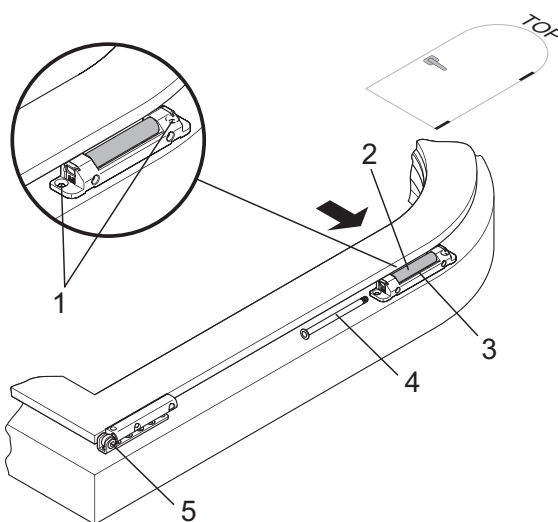
Верхняя петля Верхняя петля SWR ... для арочных окон
