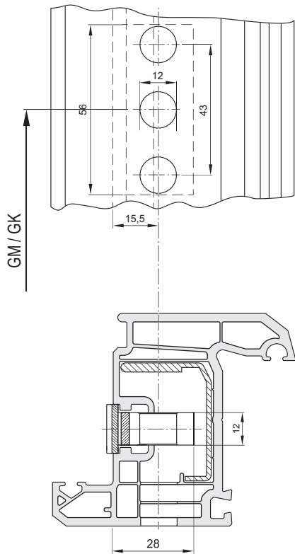
V-3-1: Сверление и фрезеровка GAK/GAM ...D = 15,5 мм
